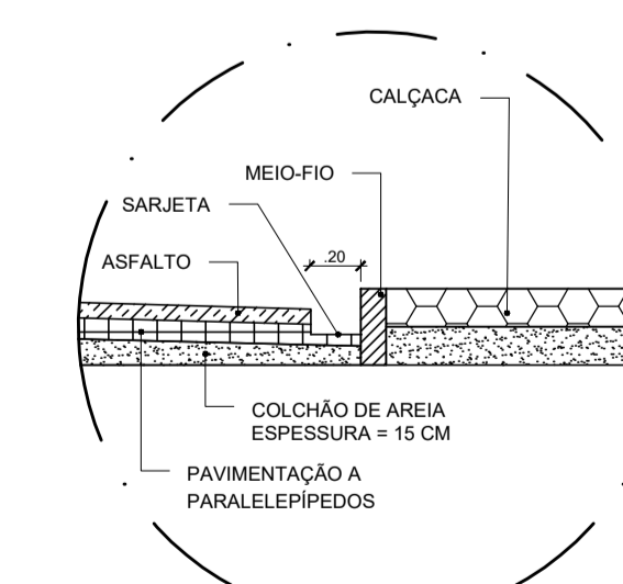
DETALHE 01 Sem Escala
