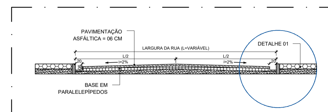
PERFIL TRANSVERSAL Sem Escala
