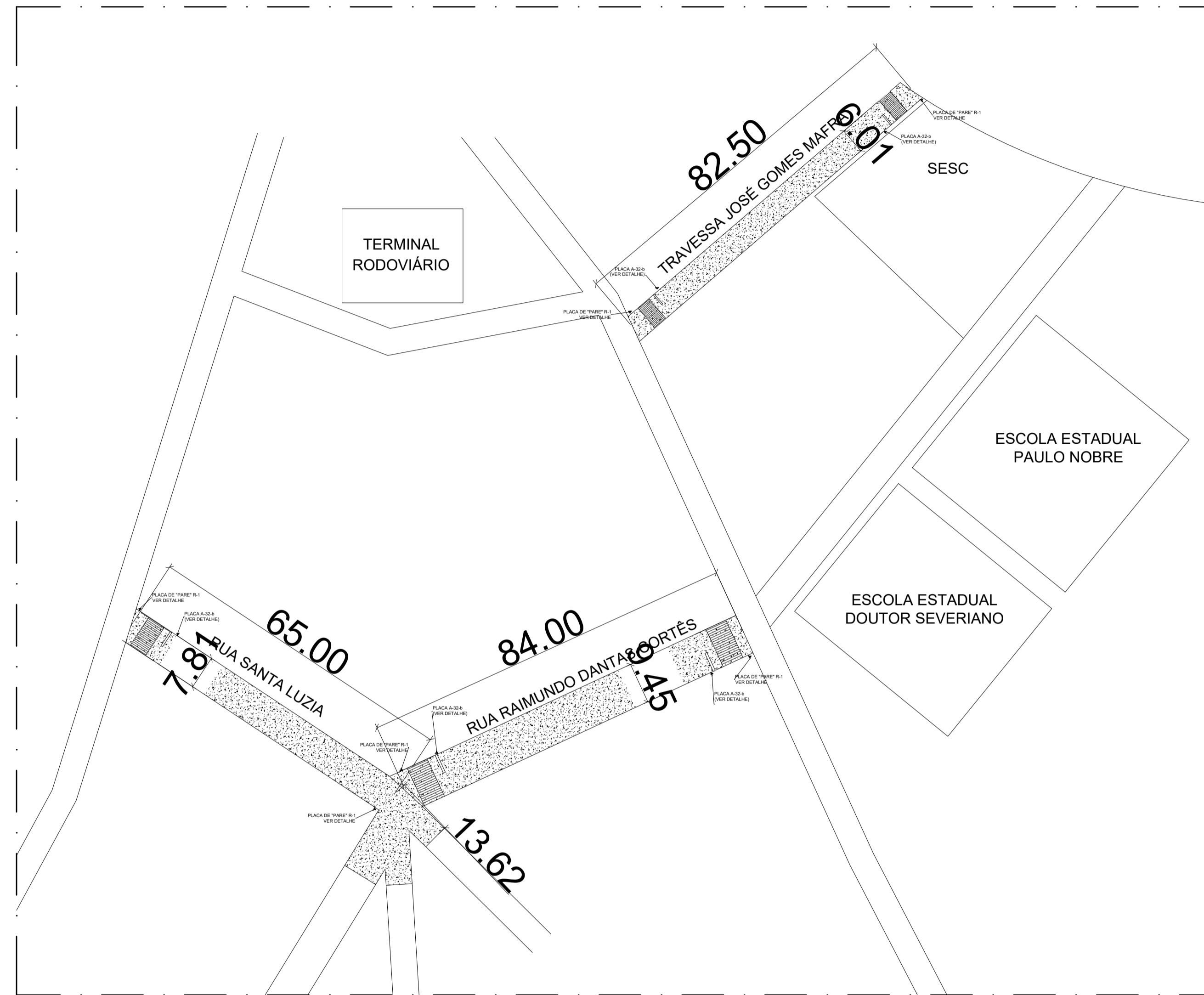
PLANTA SITUAÇÃO E LOCAÇÃO ESC: 1/750
