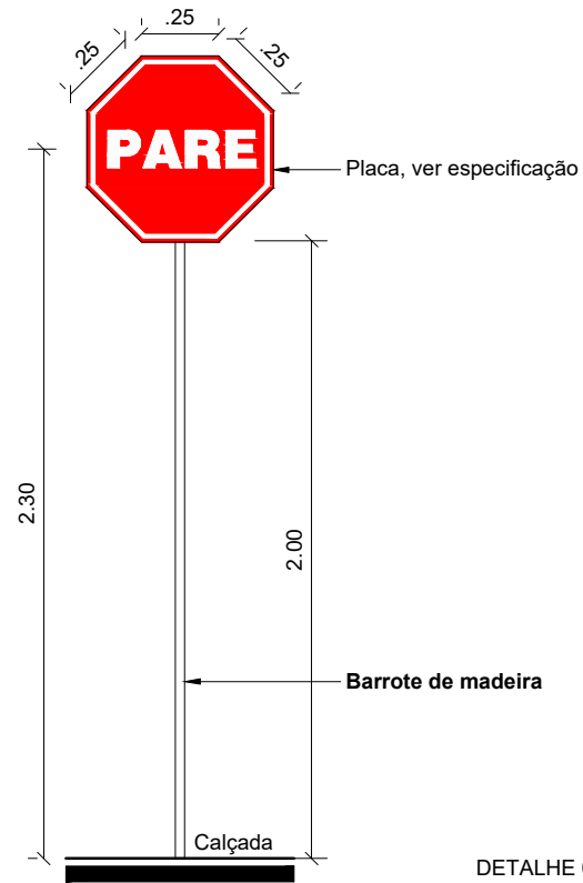
DETALHE 01 ESC: 1/25
