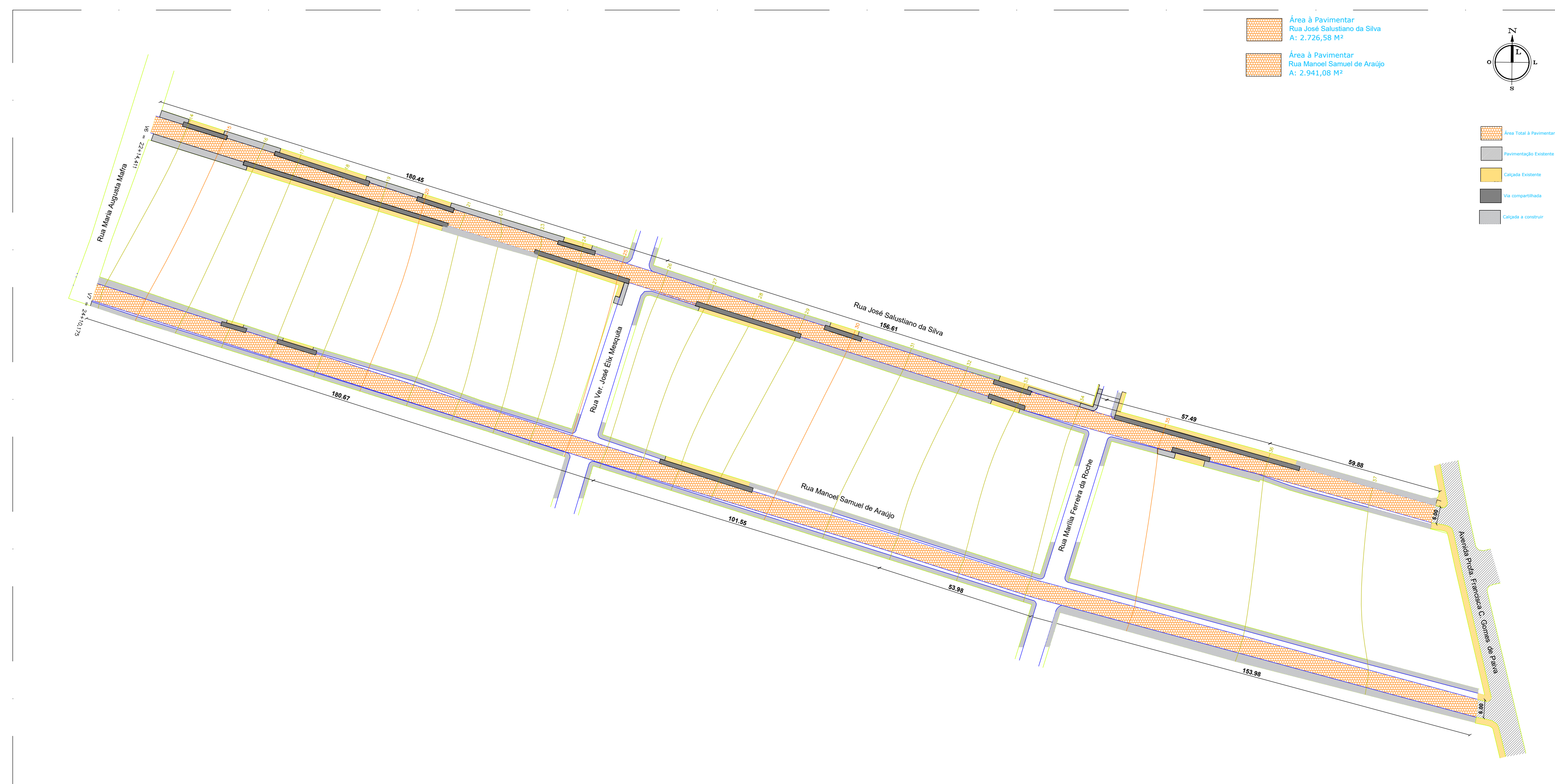
PLANTA SITUAÇÃO E LOCAÇÃO RUA JOSÉ SALUSTIANO DA SILVA E A RUA MANOEL SAMUEL DE ARAÚJO ESC.: 1/1000
