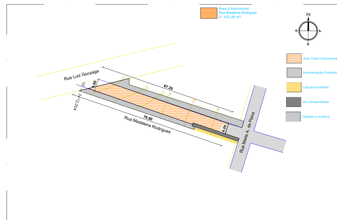
PLANTA SITUAÇÃO E LOCAÇÃO RUA MADALENA RODRIGUES ESC.: 1/1000
