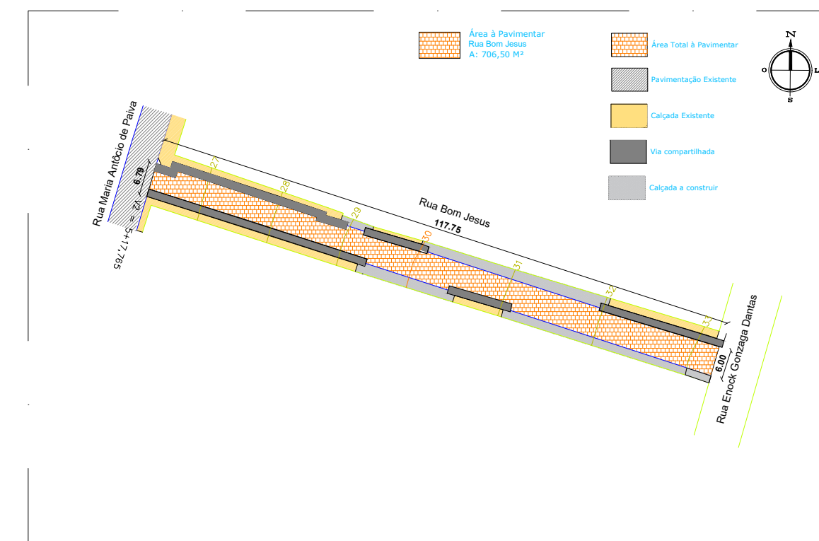
PLANTA SITUAÇÃO E LOCAÇÃO RUA BOM JESUS ESC.: 1/1000
