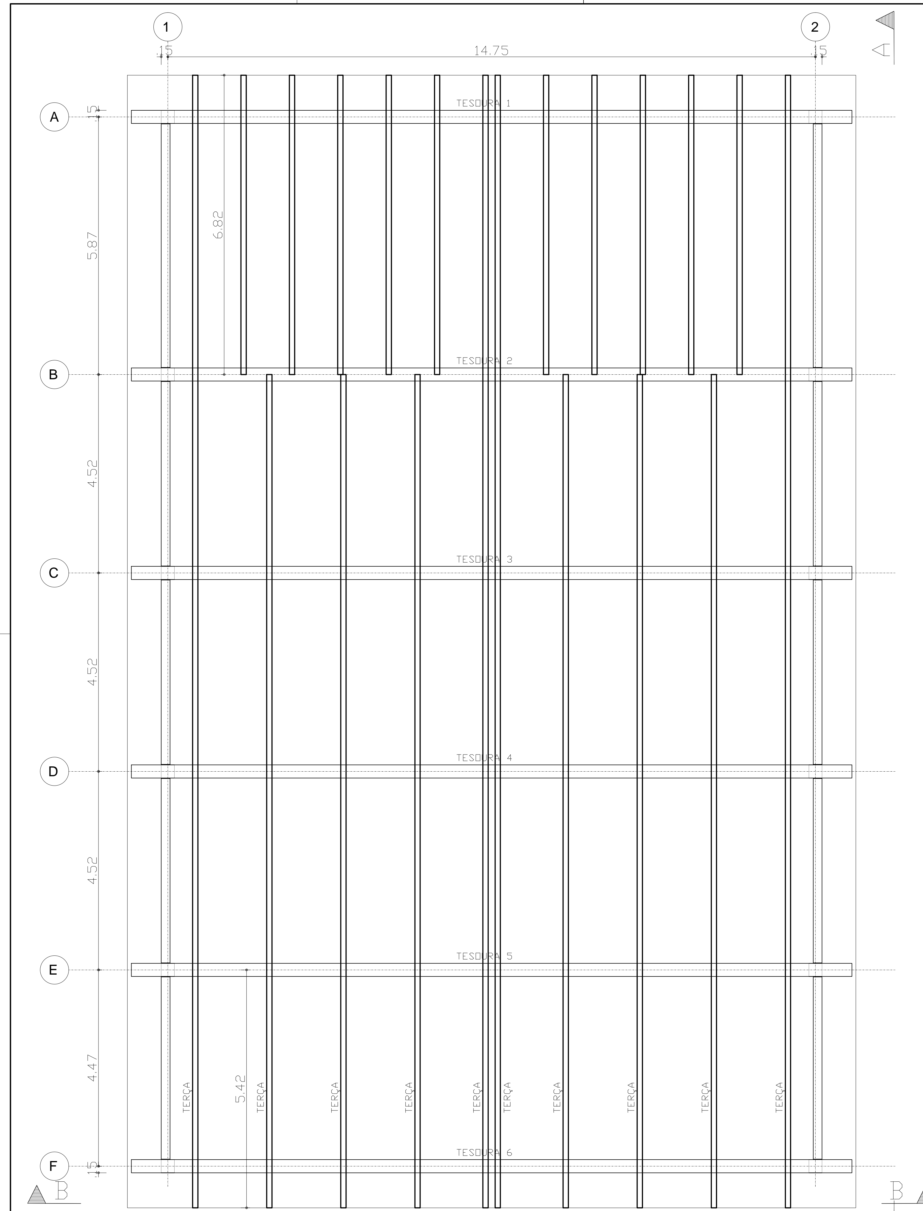
FORMA DA COBERTURA - CUMIEIRA (NÍVEL 2) ESCALA 1:50
